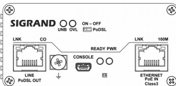
Модем SG-17B-48P/PD-M
