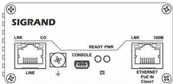
Модем SG-17B-48P-M
