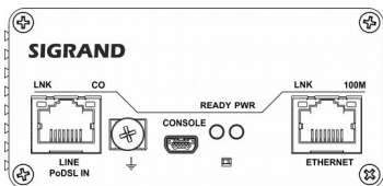
Модем SG-17B-P-M
