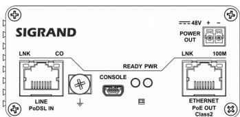
Модем SG-17B-P/T-M
