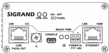
Модем SG-17B-48/PD-M
