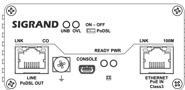
Модемы SG-17B-48P/PD-M
