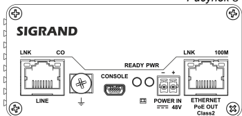
Модем SG-17B-48/T-M
