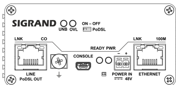
Модем SG-17B-48PD-M
